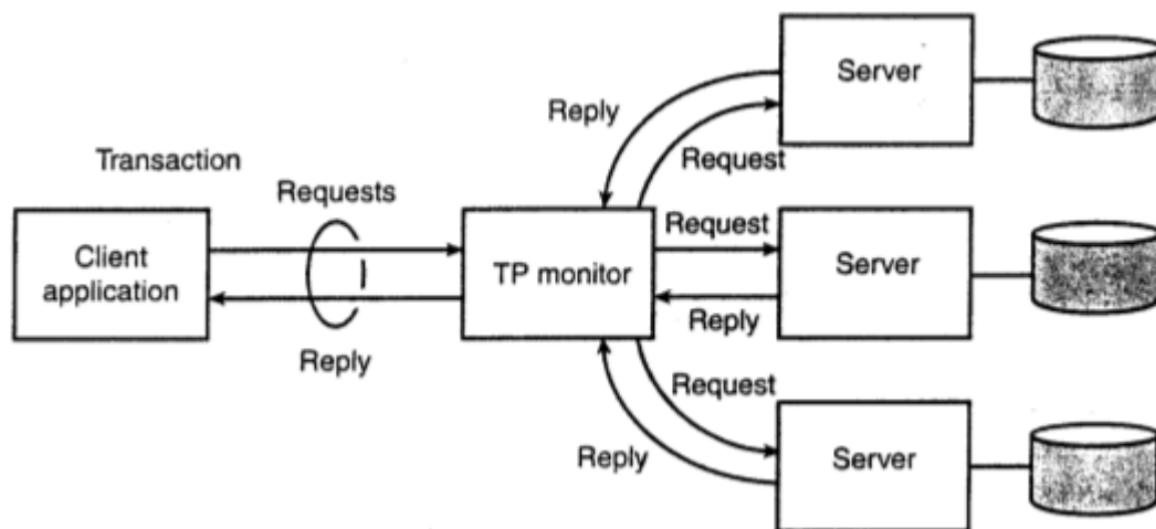
Рисунок 1. Роль монитора ТР в распределенных системах
