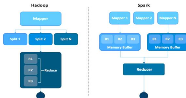
Сурет 2. Apache Hadoop және Apache Spark жүйесі
