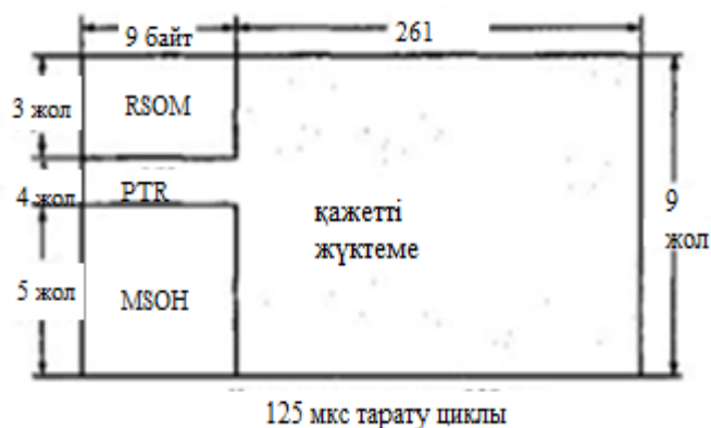
Сурет 2. STM-1 Синхронды көлік модулінің құрылымы
